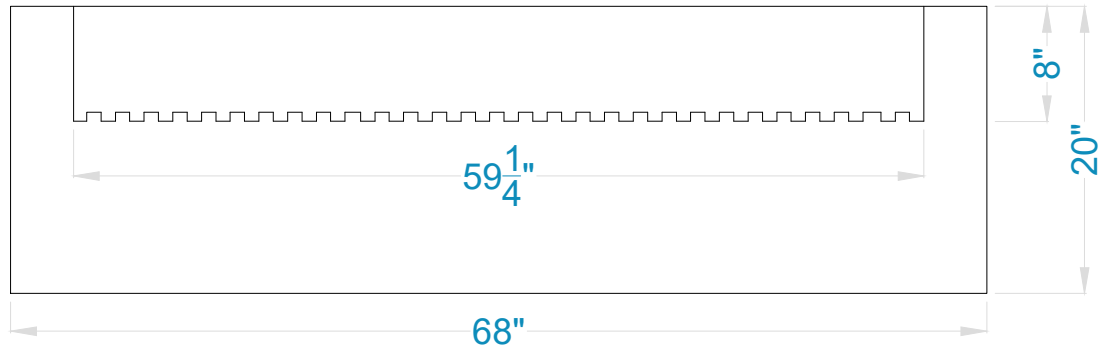
ELEVATION
